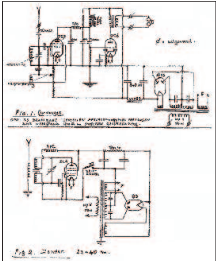
Tekening van een ontvangst- en zendinstallatie, gebouwd door enkele krijgsgevangenen in kamp Gloegoer
